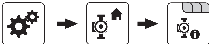
Menu Système
